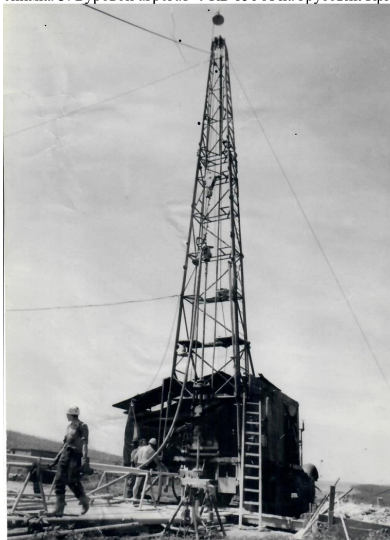
снимка 3: Буровой агрегат УКБ 650 А на грузовик КраЗ 222 ТПРП г. 1962
